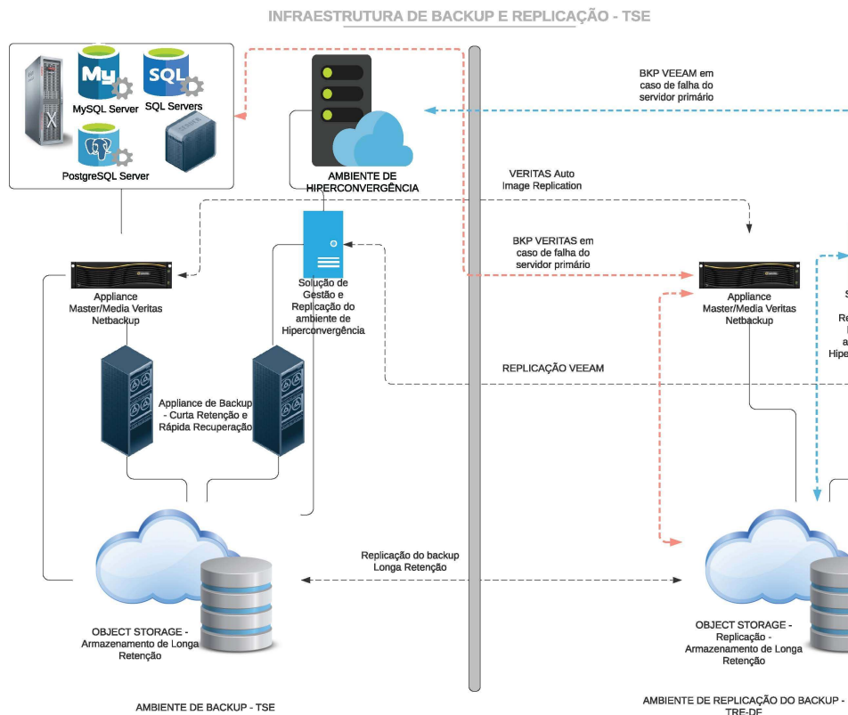
Figura 3 - Infraestrutura de Backup e Replicação
