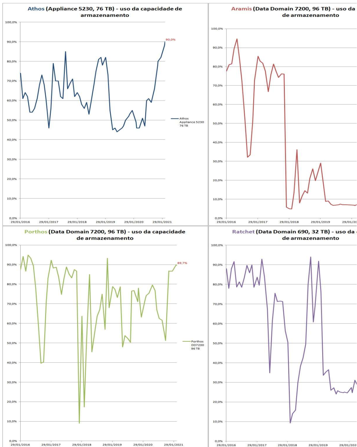
Figura 2 - Gráfico do uso da Capacidade de Armazenamento de Backup
