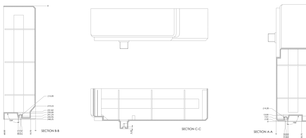
Figura 20- Medidas do encaixe lateral do dispositivo genérico
